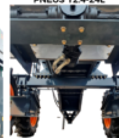
TANDEM ARTICULADO/ REGULAGEM DE BITOLA/ PNEUS 12.4-24L
