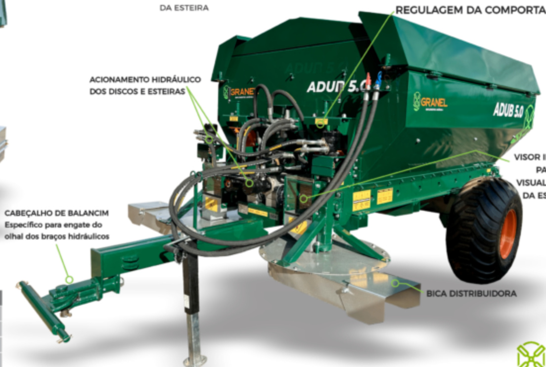
REDUTORES E VÁLVULA DE REGULAGEM DA ESTEIRA
